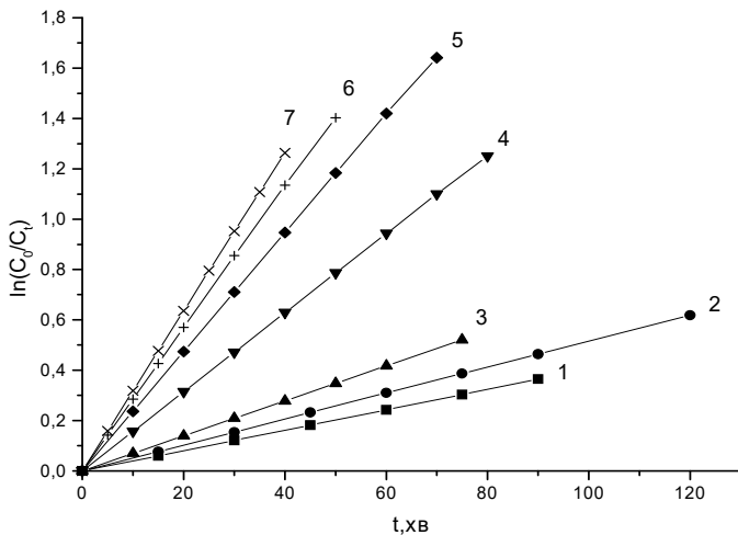
Рис. 2. Кінетичні криві реакції окиснення піридину ПДК за 318 К. Розчинник: 1 – діоксан; 2 – пропанол-2; 3 – етилацетат; 4 – толуен; 5 – ДМФА; 6 – дихлоретан; 7 – нітробензен.
